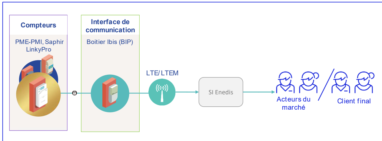
Schéma représentatif de la chaîne de transmission des données de mesure sur les domaines de tension HTA et BTSUP
